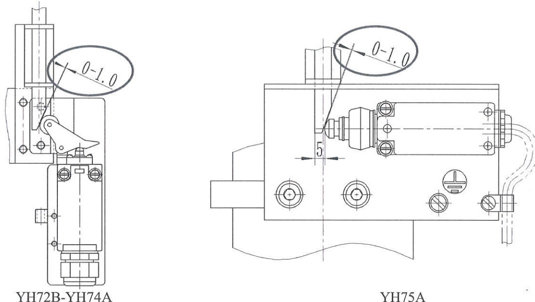
图 6 开关调整示意图
