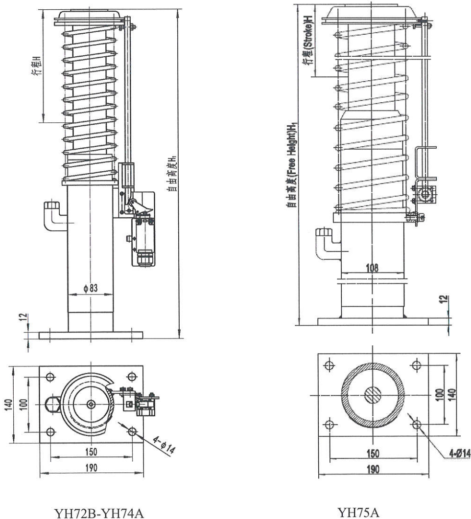
图 2 缓冲器外形图
