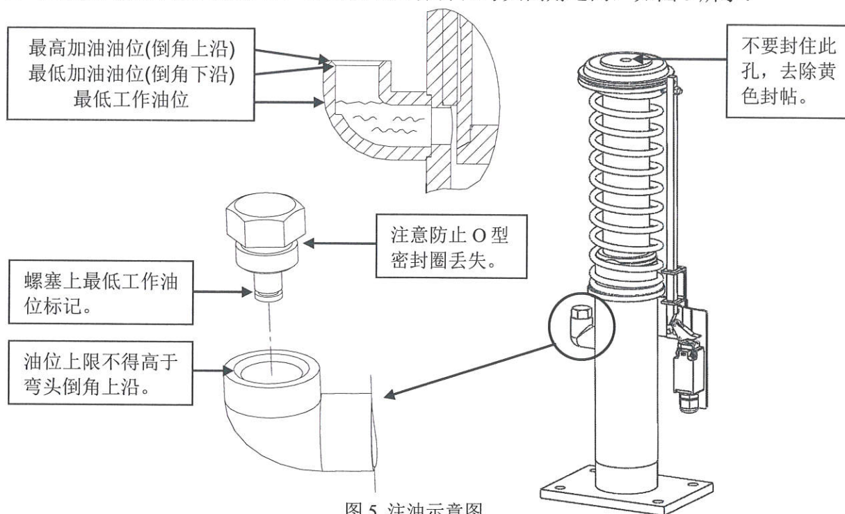
图 5 注油示意图
