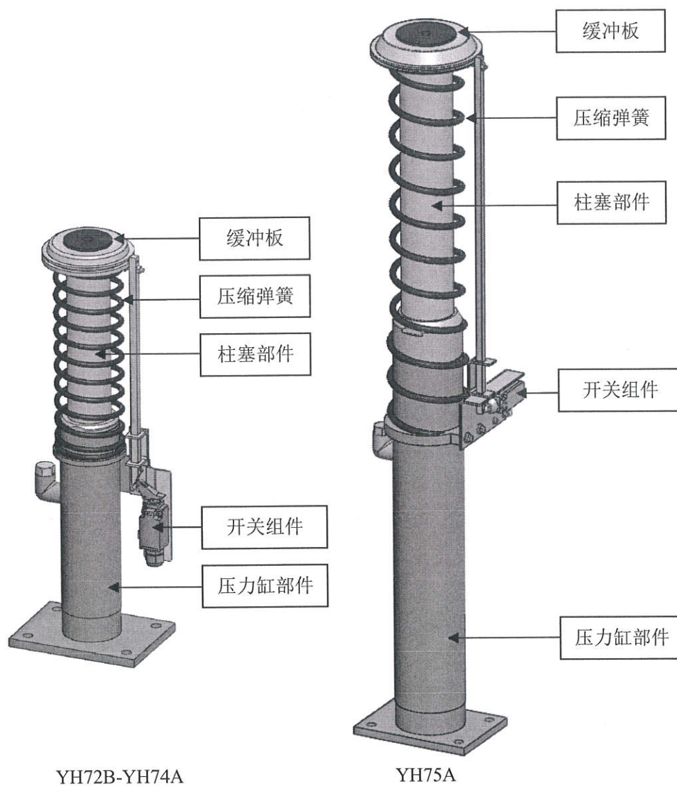
图 1 缓冲器结构示意图
