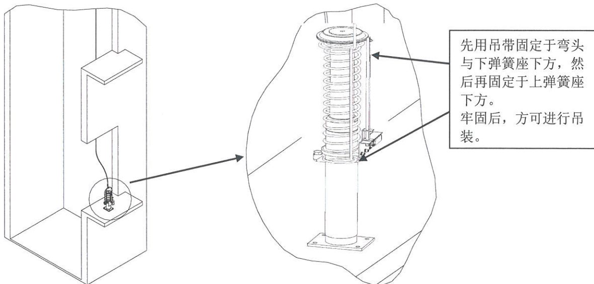
图 3 吊装示意图
