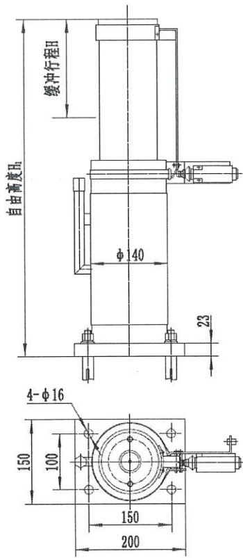
图 2 YH4、YH5 缓冲器外形图
