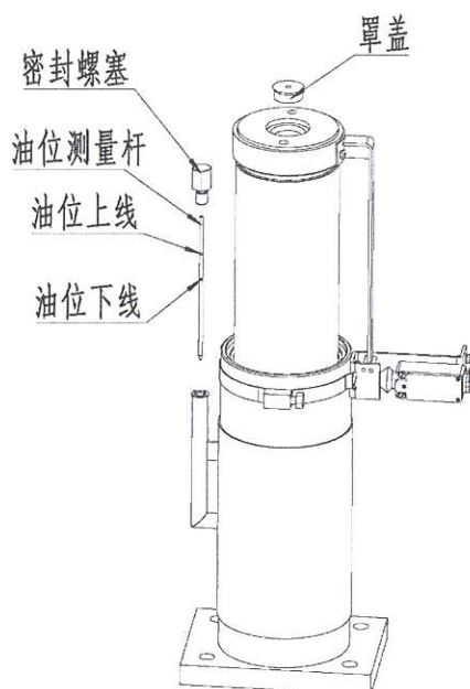
图 5 注油示意图
