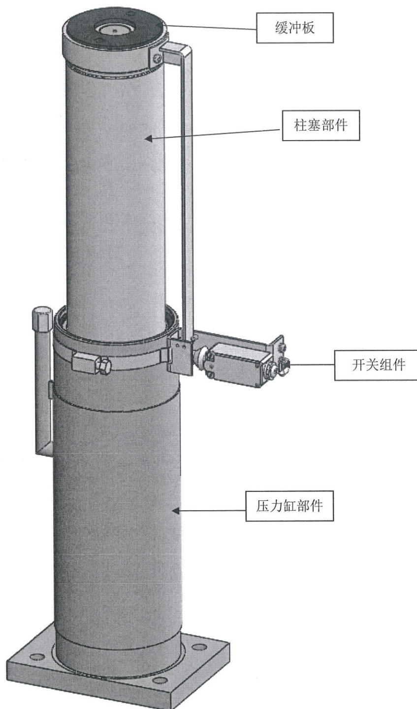
图 1 YH4、YH5 缓冲器结构示意图
