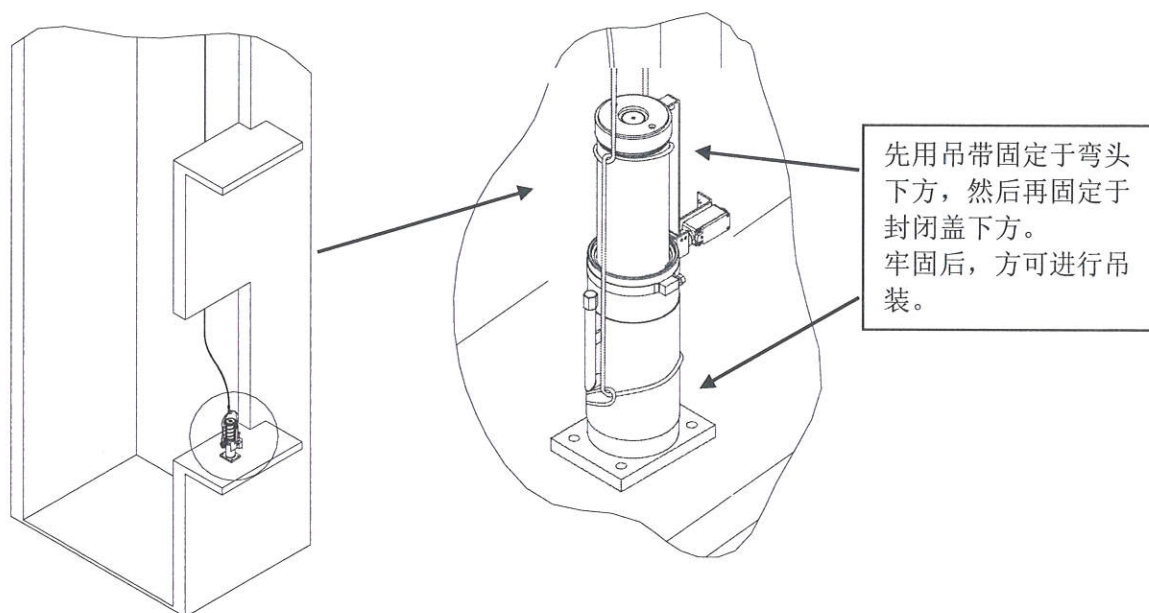
图 3 吊装示意图
