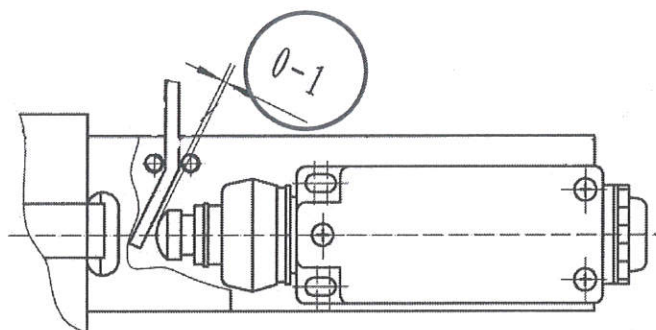
图 6 开关调整示意图
