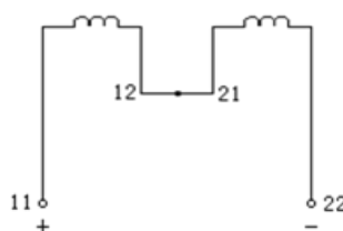
图 6-3 制动器电磁铁接线图
