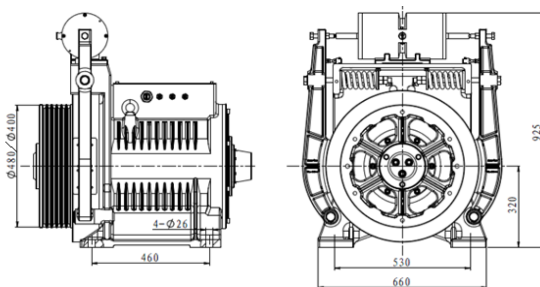
图 3-1 PMS320 曳引机（不含附件）的外形尺寸图
