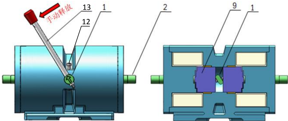
1) 释放轴 2) 推杆 9) 衔铁 12) 定位螺钉 13) 释放杆
