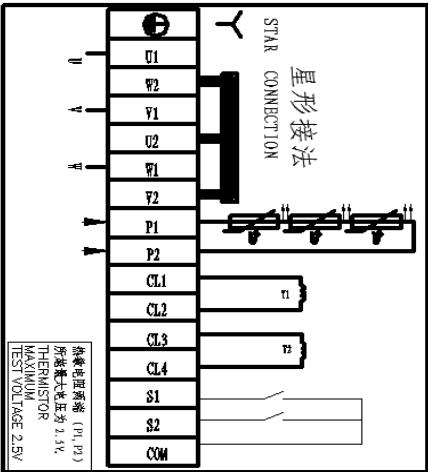
图 6-1 PMS320 曳引机接线图
