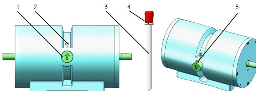
图 8-4 电磁铁组件
