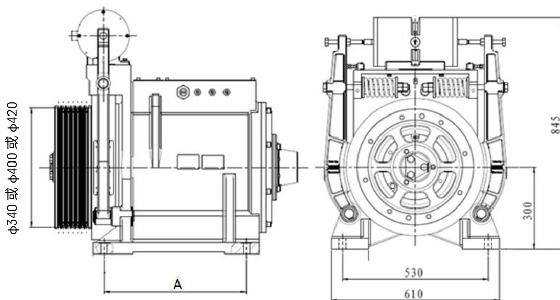
图 3-1 PMS300 曳引机（不含附件）的外形尺寸图
