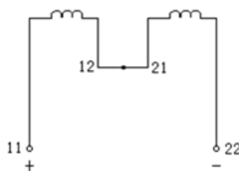
图 6-3 制动器电磁铁接线图
