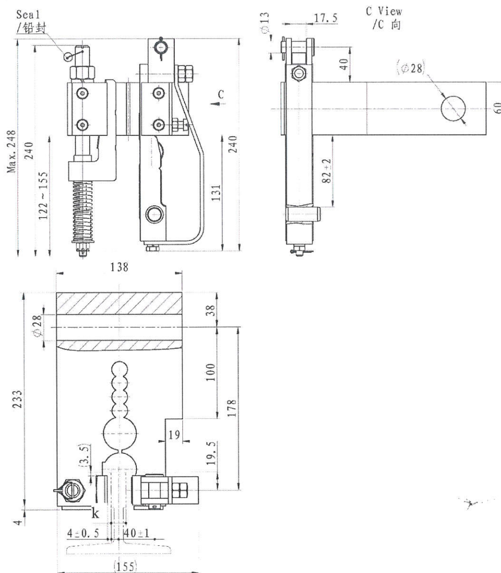
图 2 产品外形及安装尺寸示意图
