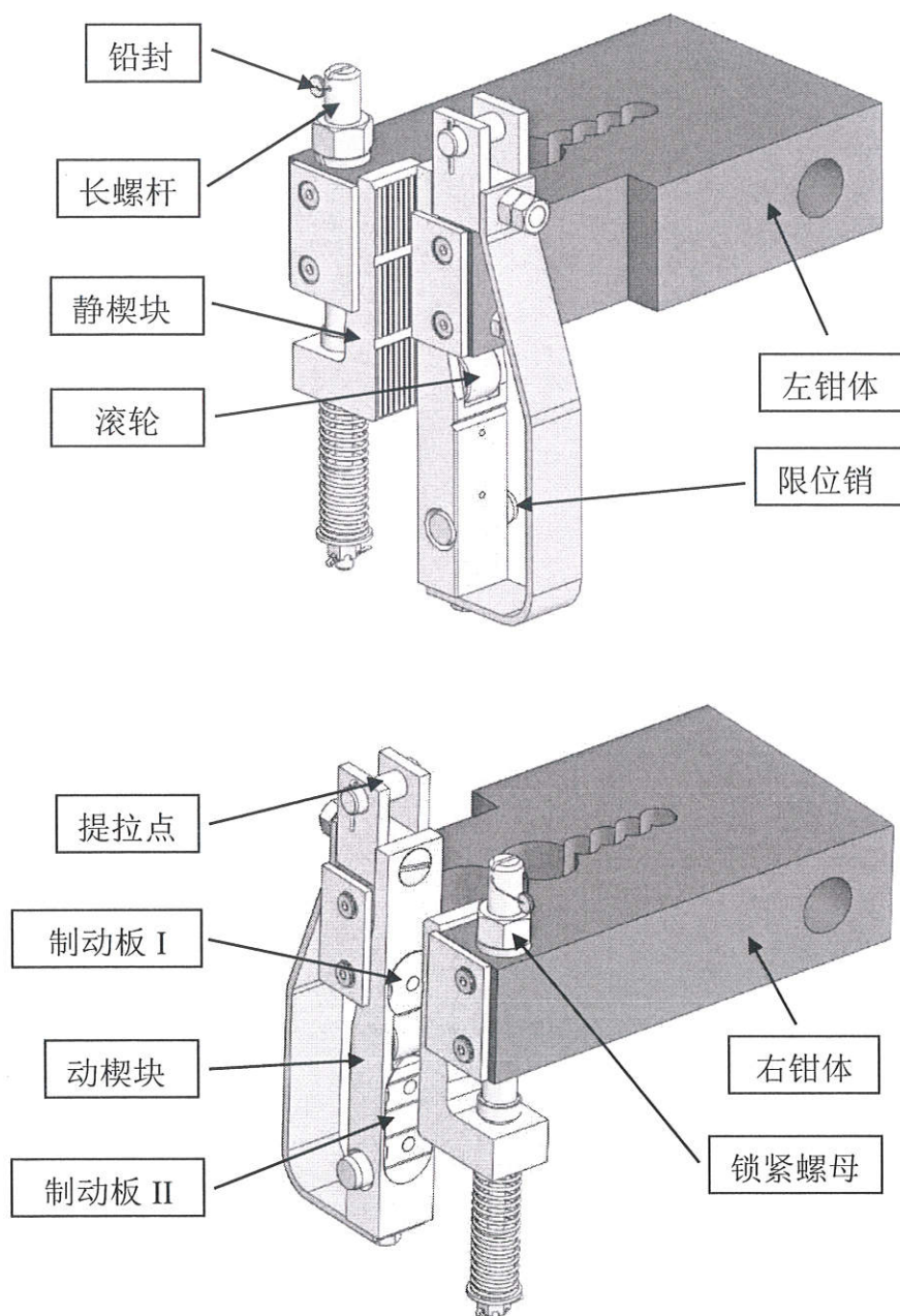
图 1 安全钳结构示意图
